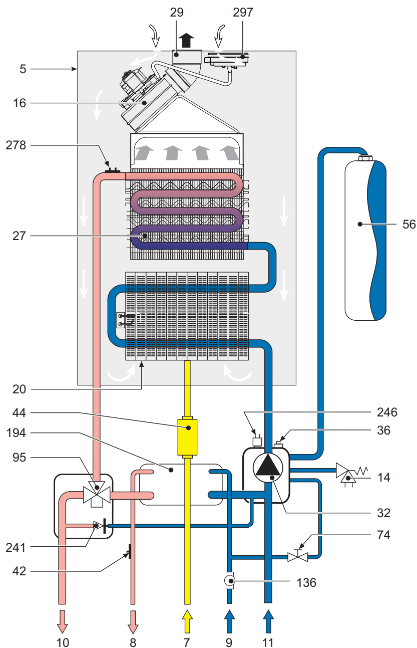
fig. 34 - Circuito idraulico
