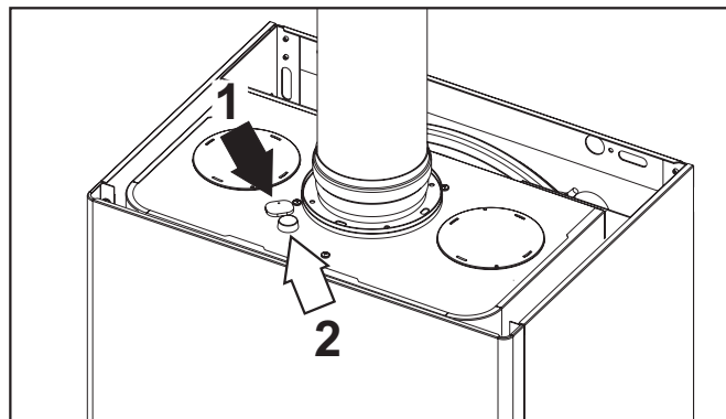
fig. 31 - Analisi fumi
